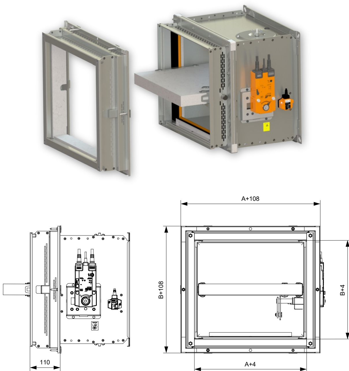
Installation frame E2
