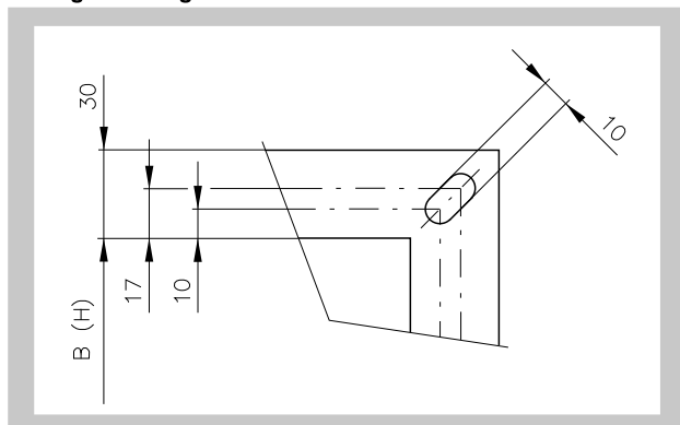
Fig. 9 Flange
