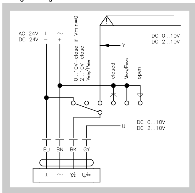
Fig. 22 Regulators GUAC-...
