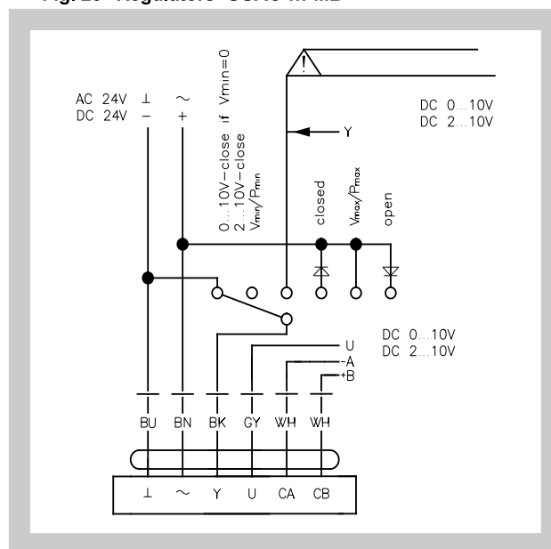
Fig. 23 Regulators GUAC-...-MB
