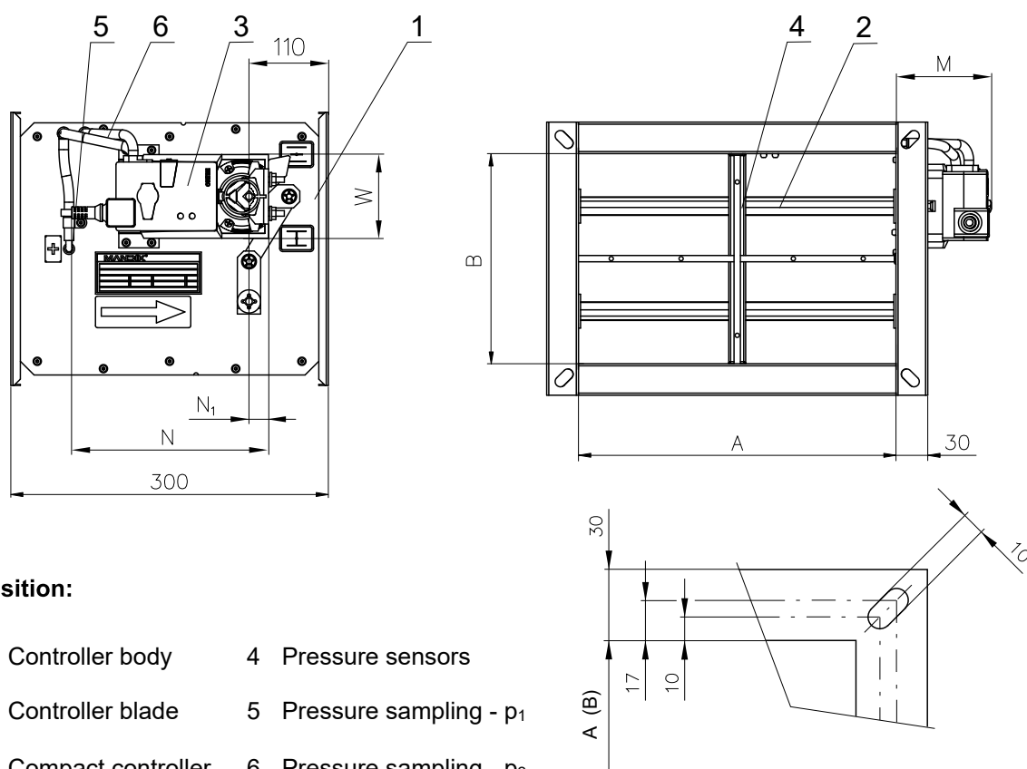
Fig. 29 RPMC-V
